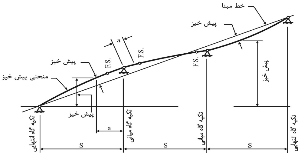
نمای جانبی پیش‌نصب تیر
