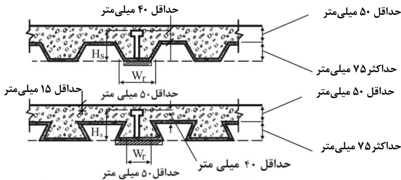
شکل ۲-۱۰-۴-۸-۲ ملاحظات و محدودیت‌های ورق‌های فولادی شکل داده شده
