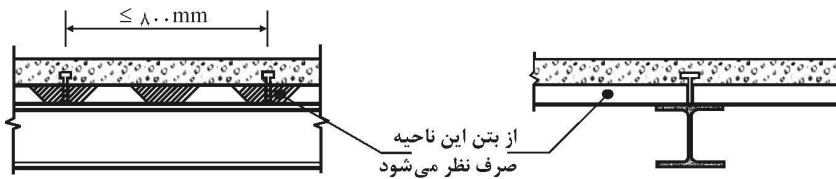
شکل ۲-۱۰-۴-۸-۵ ورق‌های فولادی شکل داده شده که کنگره‌های آنها عمود بر محور تیر می‌باشد
