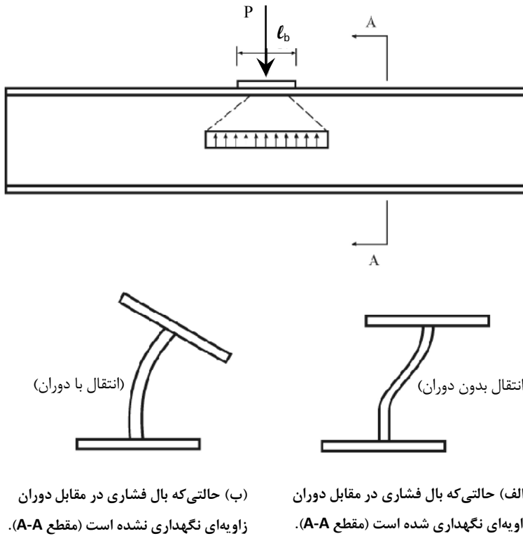
شکل ۱۰-۲-۹-۱۹ کمانش جانبی جان در مقابل نیروی متمرکز فشاری
