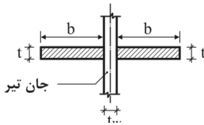
شکل ۱۰-۲-۶-۱-۱ مقطع سخت کننده های عرضی
