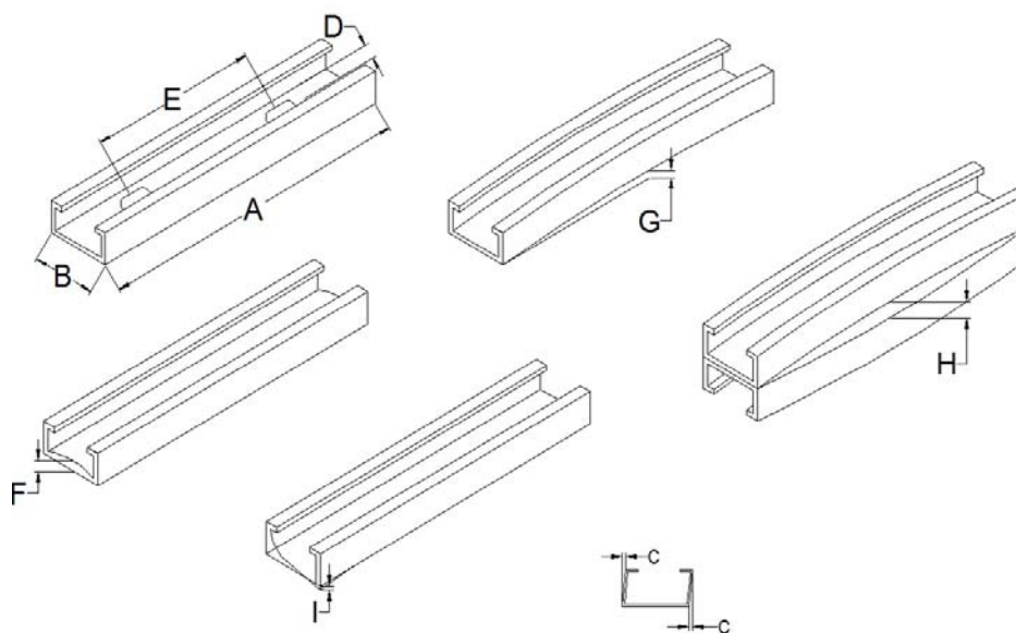
شکل ۱۱-۲-۱ رواداری ساخت اعضاء
