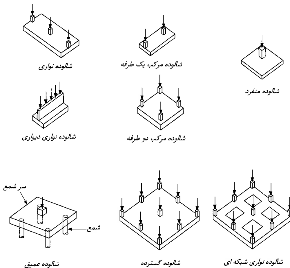
شکل ۹-۱۵-۱ انواع شالوده‌ها
