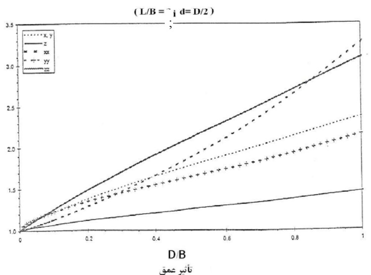
شکل (ت-۳-۴): اثرات شکل و عمق شالوده
