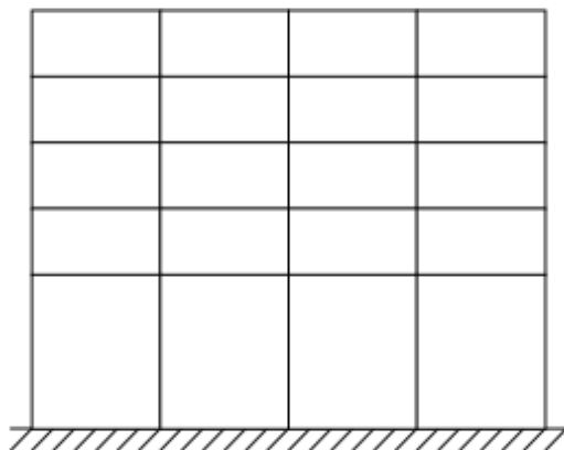
شکل ت ۱۱-۱: ساختمان با ارتفاع زیاد در طبقه اول
