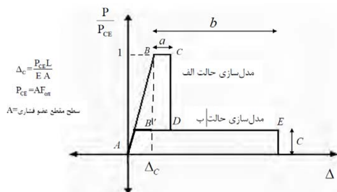
شکل (ت-۳-۵): منحنی نیرو-تغییر شکل برای مهاربند فشاری در دو حالت الف و ب
