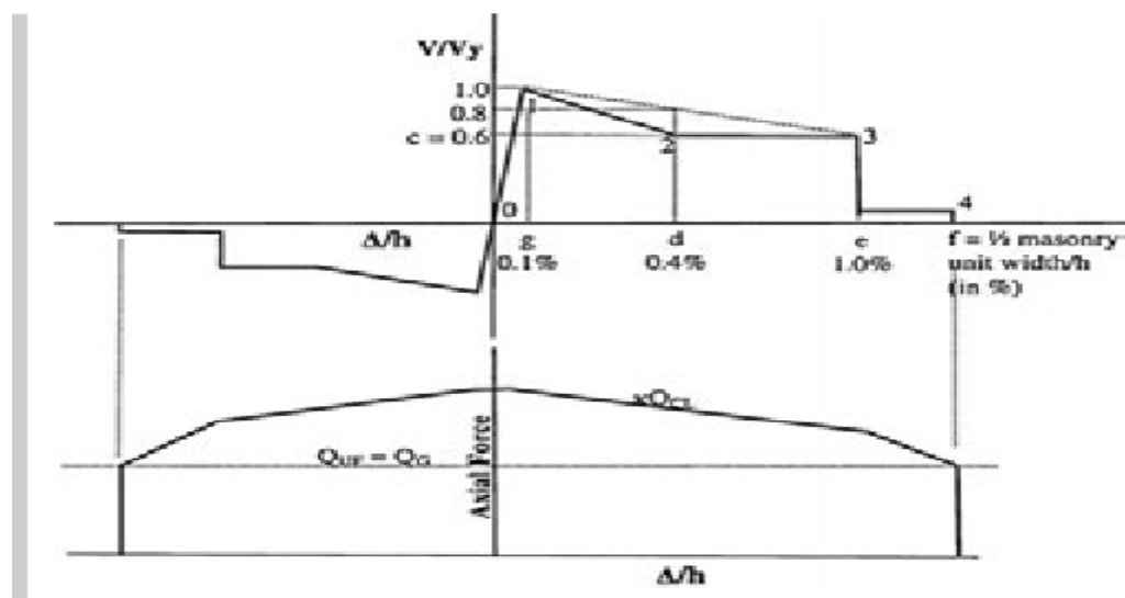
شکل ت ۷-۶-مود خرابی لغزش سطوح اتصال
