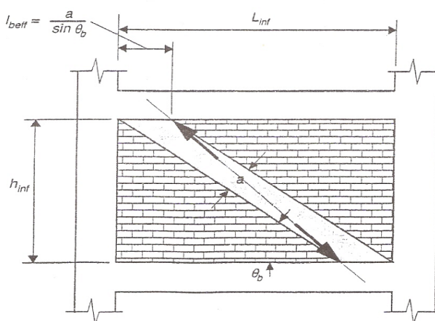
شکل (ت ۸-۷): تخمین نیروهای وارده بر تیرها
