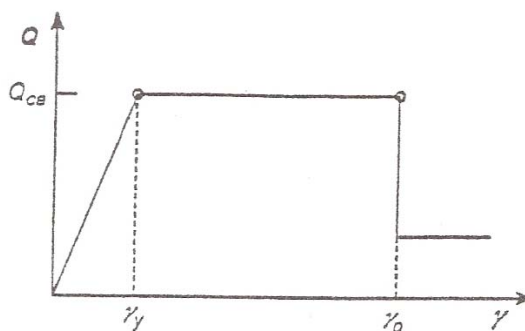
شکل (ت ۵-۸): تعریف ظرفیت تغییر شکلی تیر پیوند
