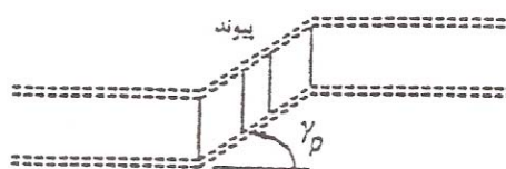
شکل (ت ۵-۷): زاویه ی چرخش تیر پیوند
