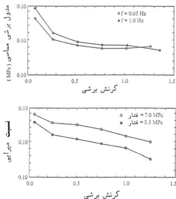
شکل (ت ۱۰-۳): مدول برشی مماسی و نسبت میرایی مؤثر تکیه‌گاه لاستیکی با میرایی زیاد
