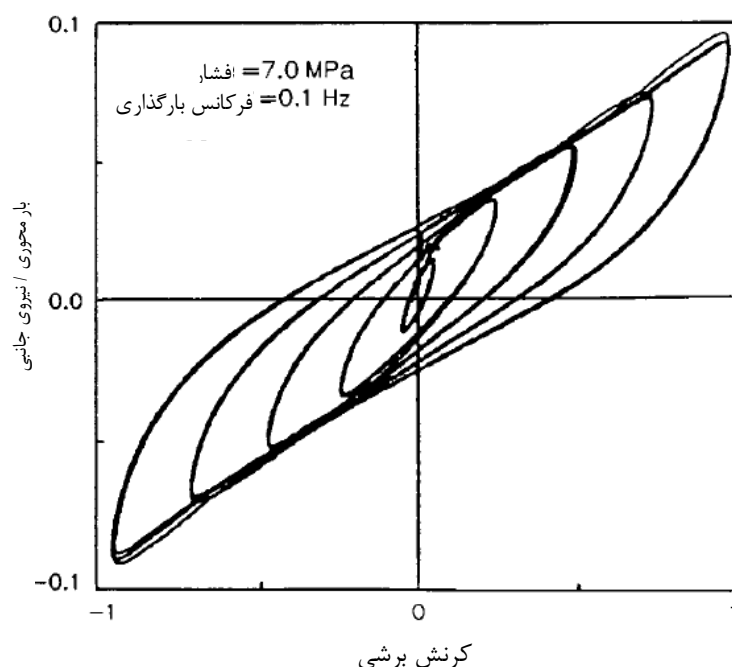
شکل (ت 10-2): حلقه‌های نیرو-تغییر مکان برای تکیه‌گاه لاستیکی با میرایی زیاد
