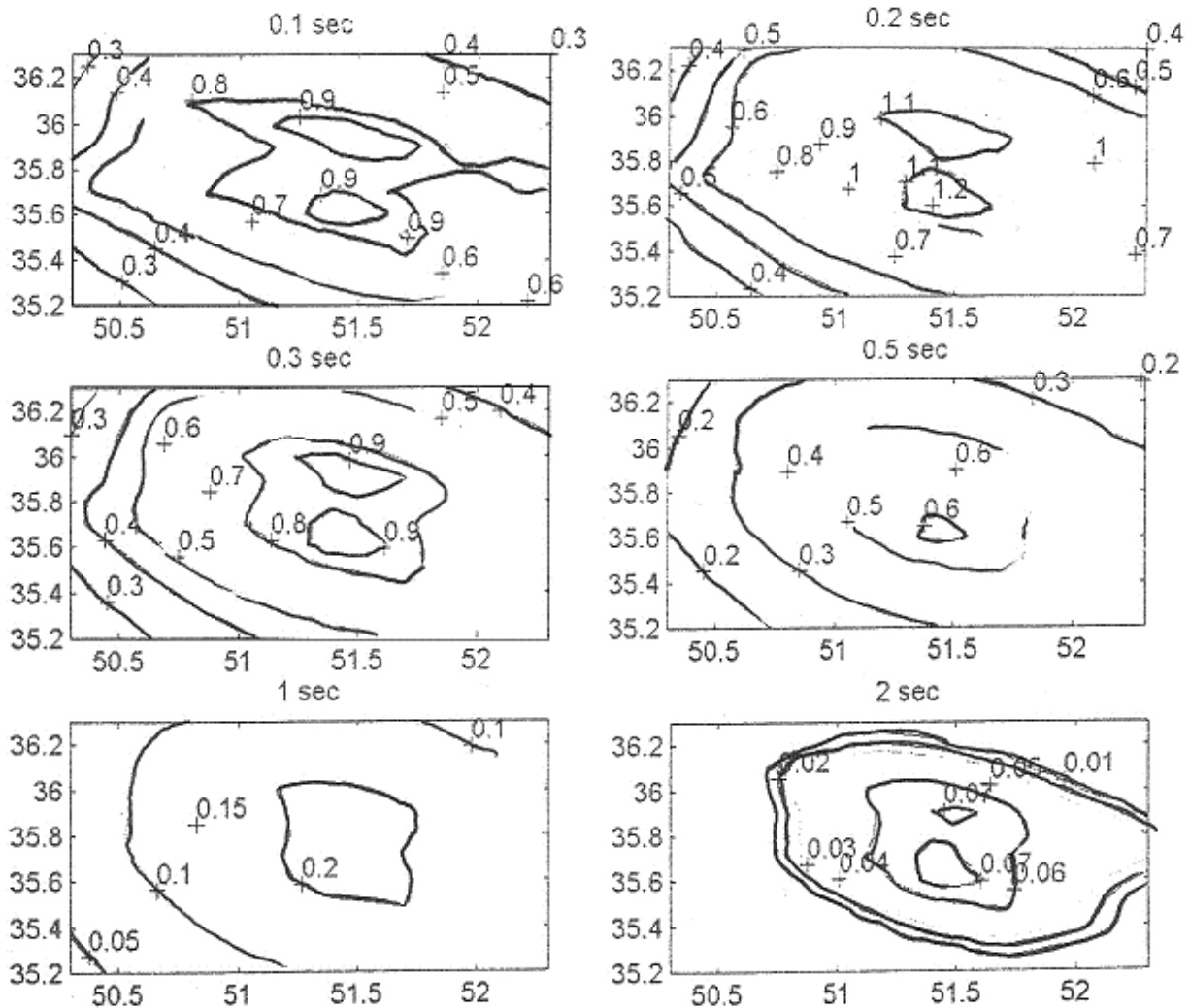
شکل (ت ۱-۵): نقشه‌های شتاب طیفی برای زمان تناوب ۰/۱، ۰/۲، ۰/۳، ۰/۵، ۱ و ۲ ثانیه برای ناحیه تهران
