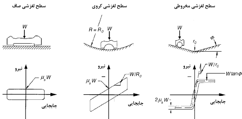
شکل (ت 10-5): حلقه‌های نیرو - جابجایی تکیه‌گاه‌های لغزشی
