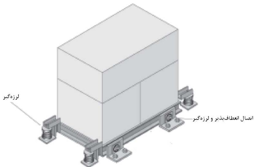
شکل ۱-۷-۲۱-۲- اتصال تجهیز با استفاده از اتصالات انعطاف‌پذیر و لرزه‌گیر
