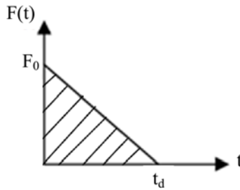
شکل ۲۱-۵-۲- تغییرات بار انفجاری روی سازه یک درجه آزادی
