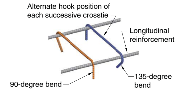
Fig. R25.3.5—Crosstie.
